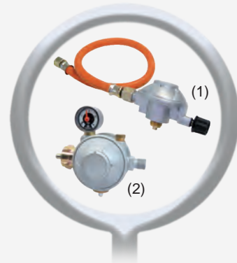
(1) Sicherheitsadapter R mit Druckminderer und DVGW- Schlauch (0,5 m), für Flaschen R 901 / R 904 / R 907 Art.-Nr. 6.000.840
