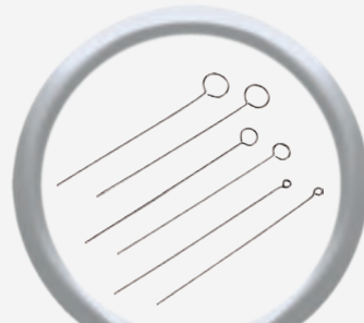
Impfösen , Draht Ø 0,6 mm Spezial-Edelstahl Ø 1 mm Art.-Nr. 6.000.371 Ø 3 mm Art.-Nr. 6.000.373 Ø 5 mm Art.-Nr. 6.000.375 Platin / Iridium Ø 1 mm Art.-Nr. 6.000.381 Ø 3 mm Art.-Nr. 6.000.383 Ø 5 mm Art.-Nr. 6.000.385
